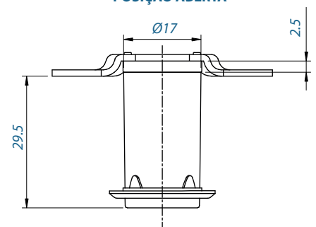
POSIÇÃO ABERTA
