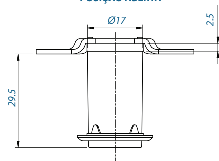
POSIÇÃO ABERTA
