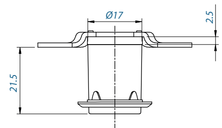
POSIÇÃO ABERTA
